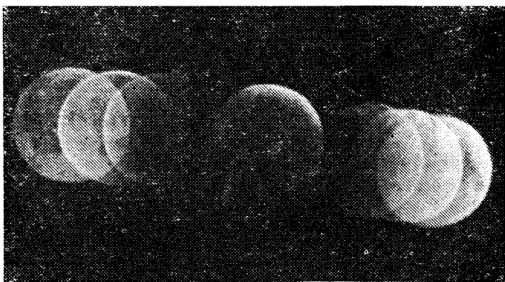
Рис. 56. Полное лунное затмение 29 ноября 1974 г. Японский любитель Акира Фуджи сделал этот выразительный снимок объективом с фокусным расстоянием 300 мм. Луна движется справа налево. Частные фазы с выдержкой 1/60 с, полная — с выдержкой 3 мин
