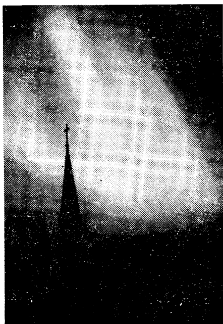
Рис. 45. Красное полярное сияние над Гарвардской обсерваторией 18 сентября 1941 г. Выдержка 10 с. Фото Р. Мэйолла
