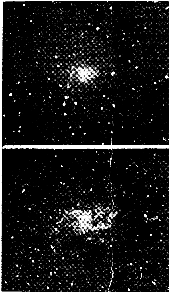
Рис. 78. Галактика М 33, как ее показывают 150-миллиметровый рефлектор (а) и «Танр-3» (б). Первая фотография получена на пленке «А-500» за 30 мин, вторая на пленке «Фото-130» за 40 мин. Фото Л. Л. Сикорука
