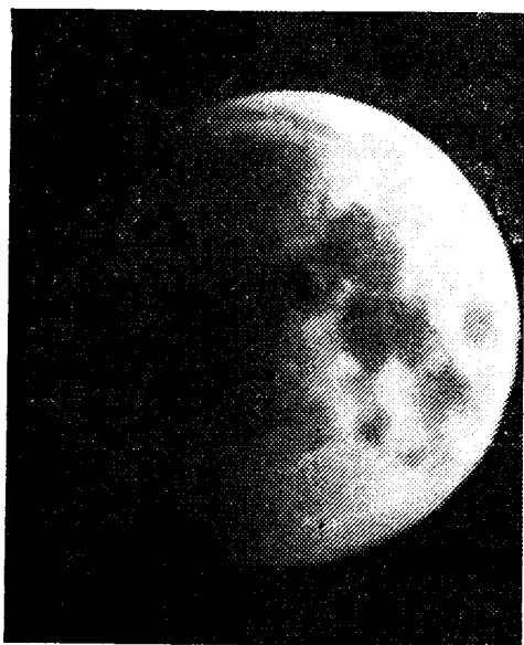
Рис. 51. Лунное затмение 16 сентября 1978 г. Перед «Зенитом-В» (объектив «Гелиос-44») была укреплена подзорная труба с увеличением 20 \times . Пленка «Фото-130», выдержка 1/30 с. Фото Л. Л. Сикорука
