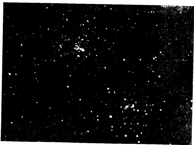
Рис. 75. Скопление h и \chi Персея на снимке Л. Л. Сикорука с рефлектором. Хотя здесь подробностей видно больше, предыдущий снимок выглядит выразительнее.
