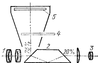
Рис. 37. Окулярная камера с расщепляемым лучом: 1 — проекционный объектив, 2 — призма Дове, 3 — окуляр визира, 4 — затвор, 5 — фотопластинка
