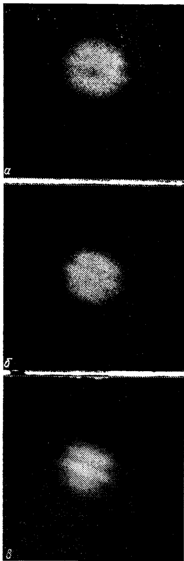
Рис. 67. Юпитер в августе 1985 г. 150-миллиметровый рефлектор Ньютона, A_{\text{эки}}=1.80 , выдержка 1/2 с. Даны отпечаток с одного негатива (а), отпечаток с трех негативов (б) и отпечаток с двенадцати негативов (в). Фото Л. Л. Сикорука
