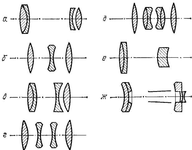
Рис. 16. Некоторые объективы, применяемые в любительской астрофотографии: «Петцваль» (а), «Триплет» (б), «Тессар» («Индустар») (в), «Ортогвоз» (объектив Росса) (г), «Гелиос» (д), «Таир» (е), «МТО-1000» (ж)
